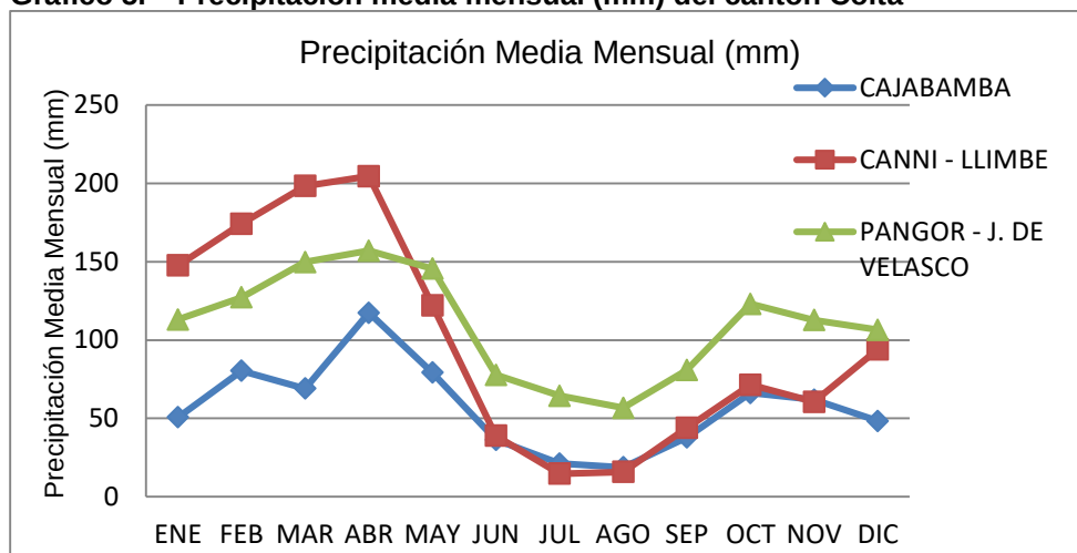
Gráfico 5. Precipitación media mensual (mm) del cantón Colta
