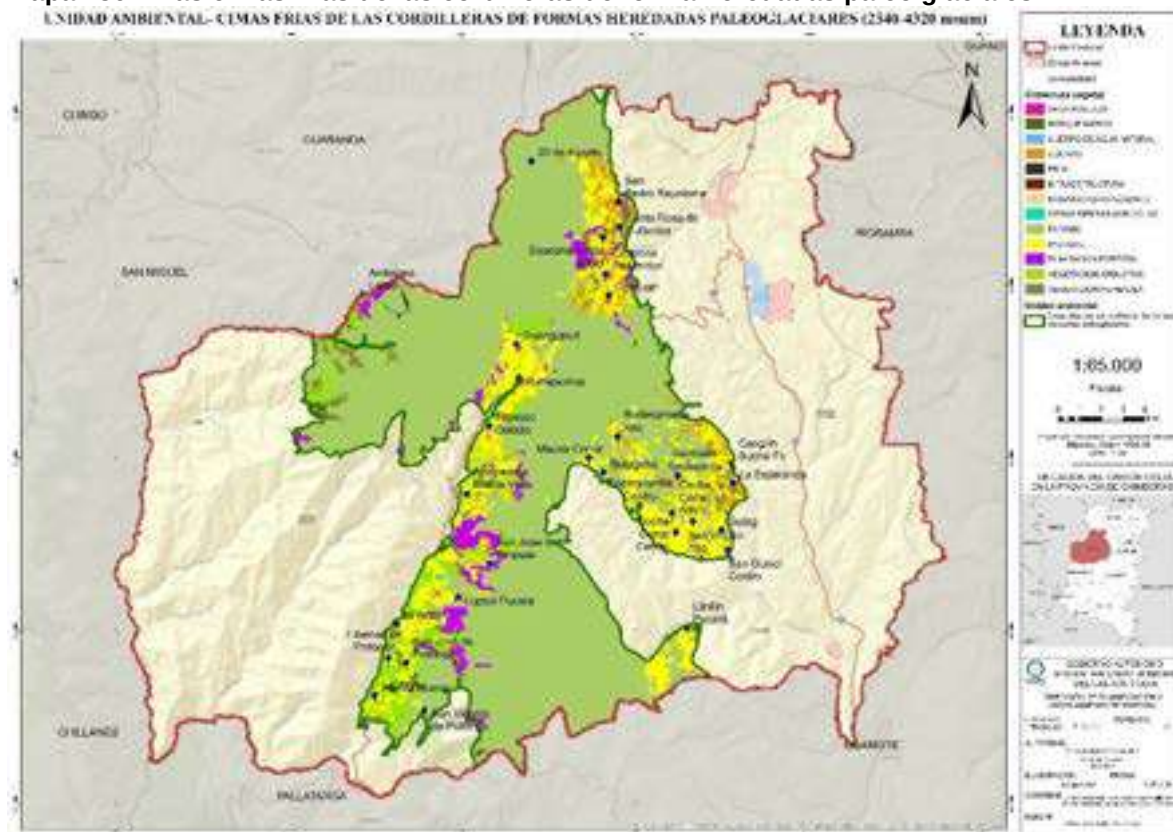
Mapa 136. Las cimas frías de las cordilleras de forma heredadas paleo glaciares
