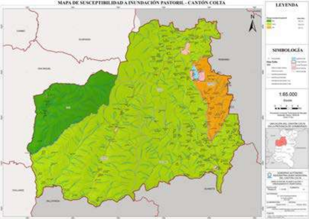
Mapa 21. Mapa de susceptibilidad a inundación pastoril cantón Colta
