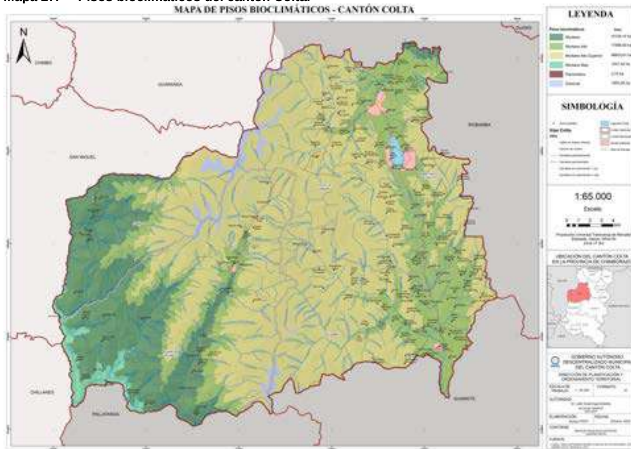
Mapa 27. Pisos bioclimáticos del cantón Colta.
