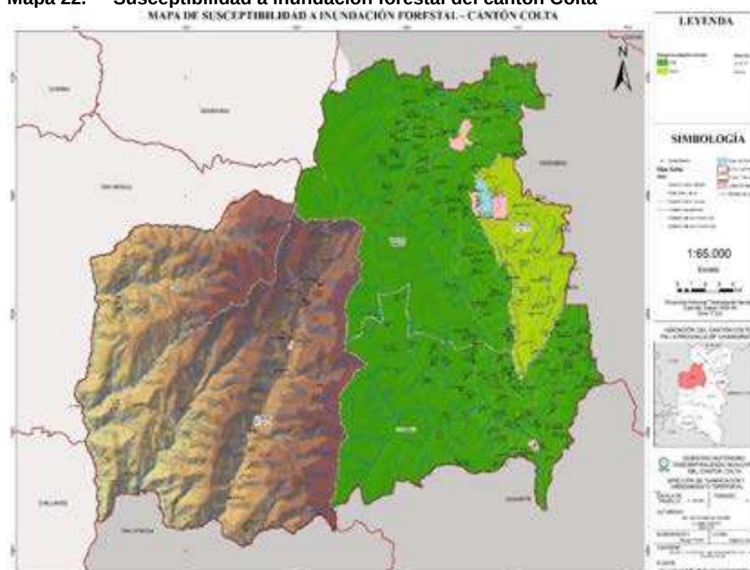
Mapa 22. Susceptibilidad a inundación forestal del cantón Colta
